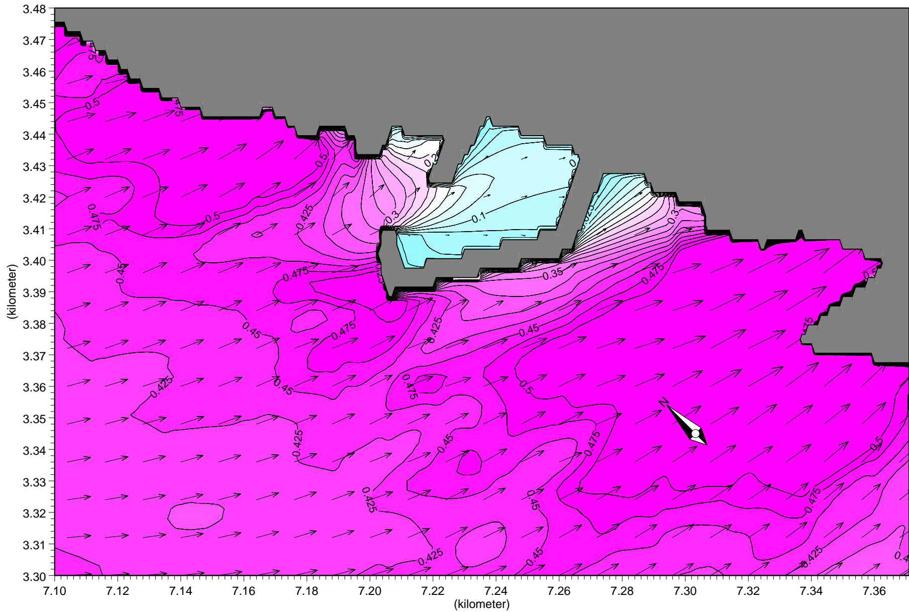
Joonis 7 Lained loodetuulega Pikendatud välismuul
