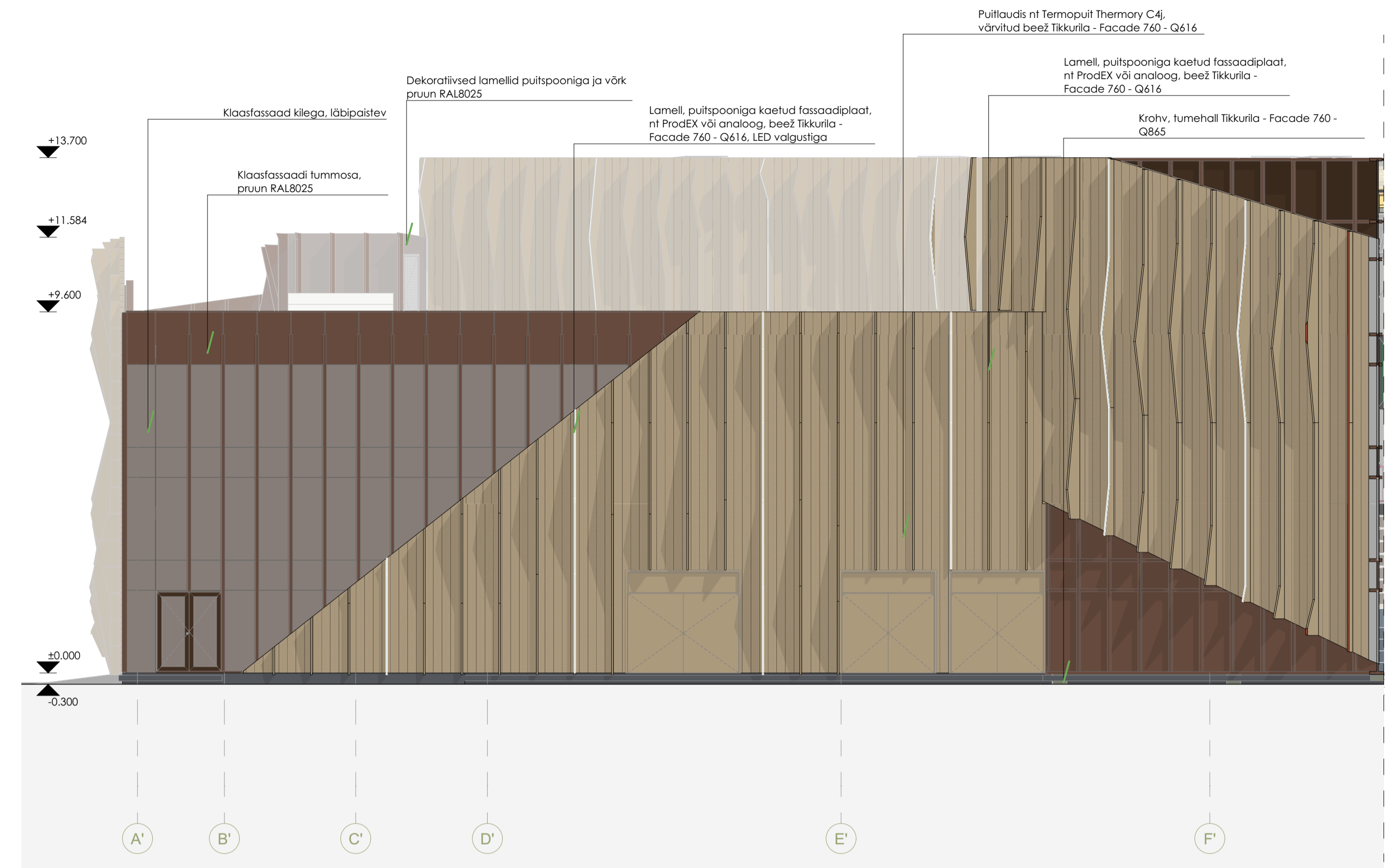
Vaade A
