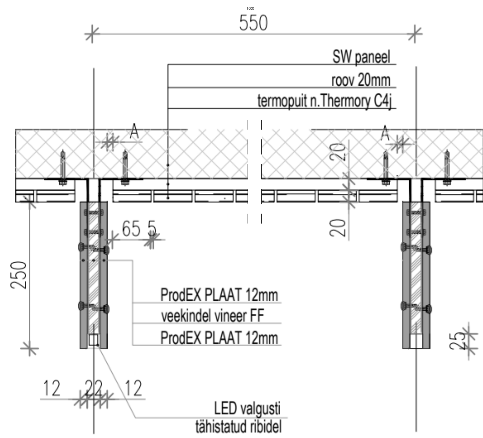
Fassaadi talade sõlm
